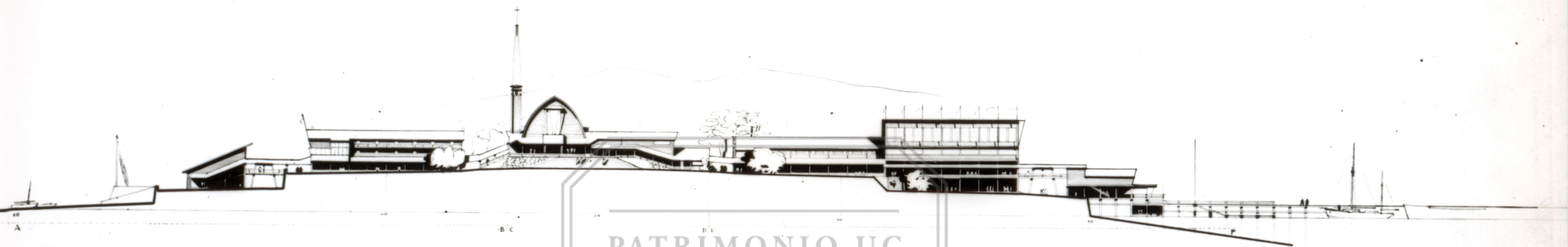
ELEVACION GENERAL GRAN PLAZA
