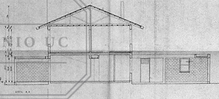
CORTE A-A
