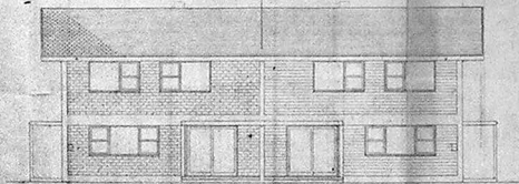
ELEVACION POSTERIOR
