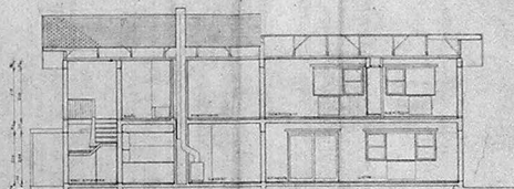
CORTE A-B
