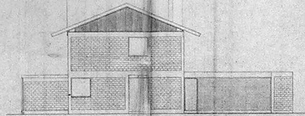
ELEVACION LATERAL
