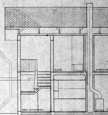
CORTE B-B
