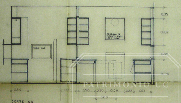
CORTE AA
