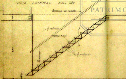
VISTA LATERAL ESC. 1:20
