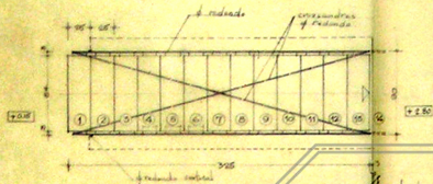
VISTA LATERAL ESC. 1:20
