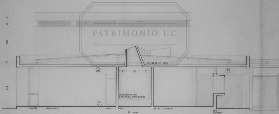
CORTE TRANSVERSAL C C
