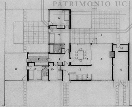
PLANTA PRIMER PISO
