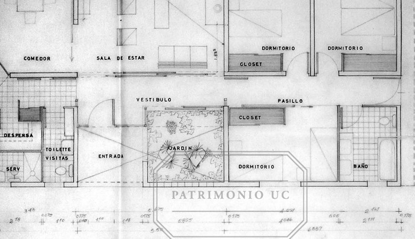
PLANO DE PLANTA
