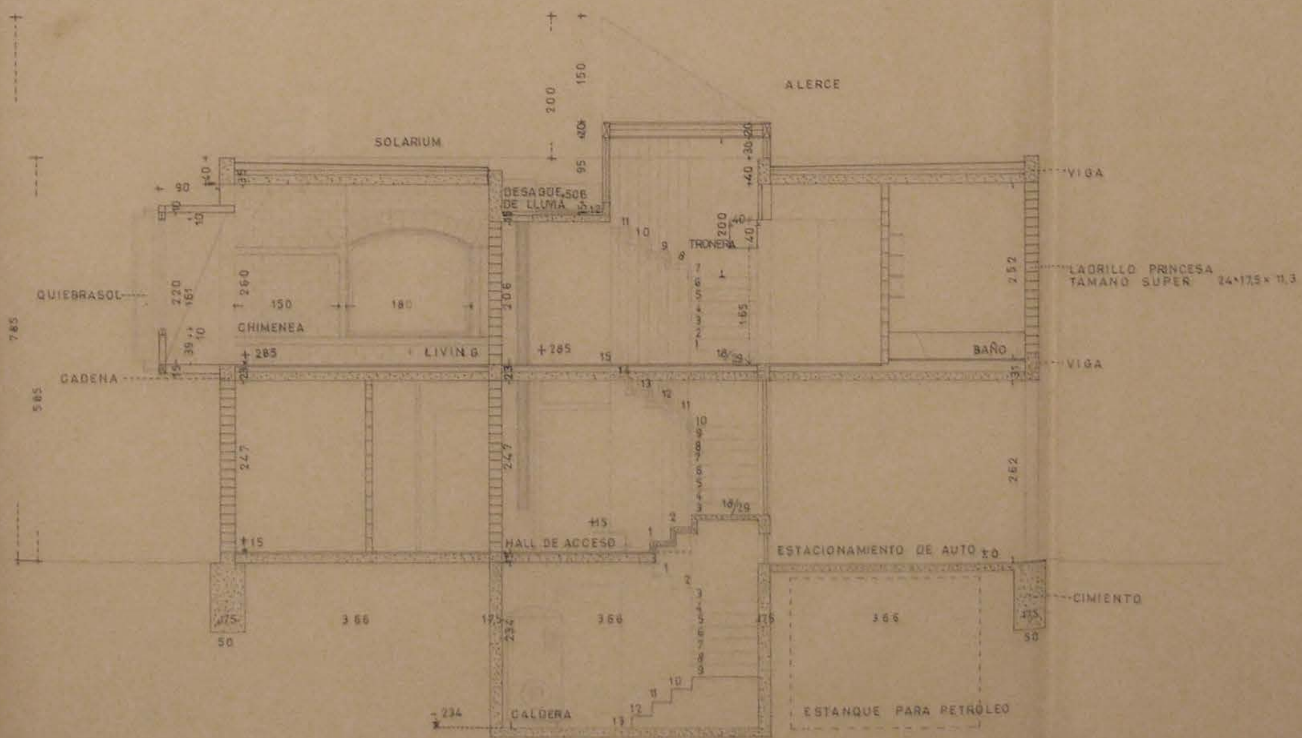
CORTE A-A
