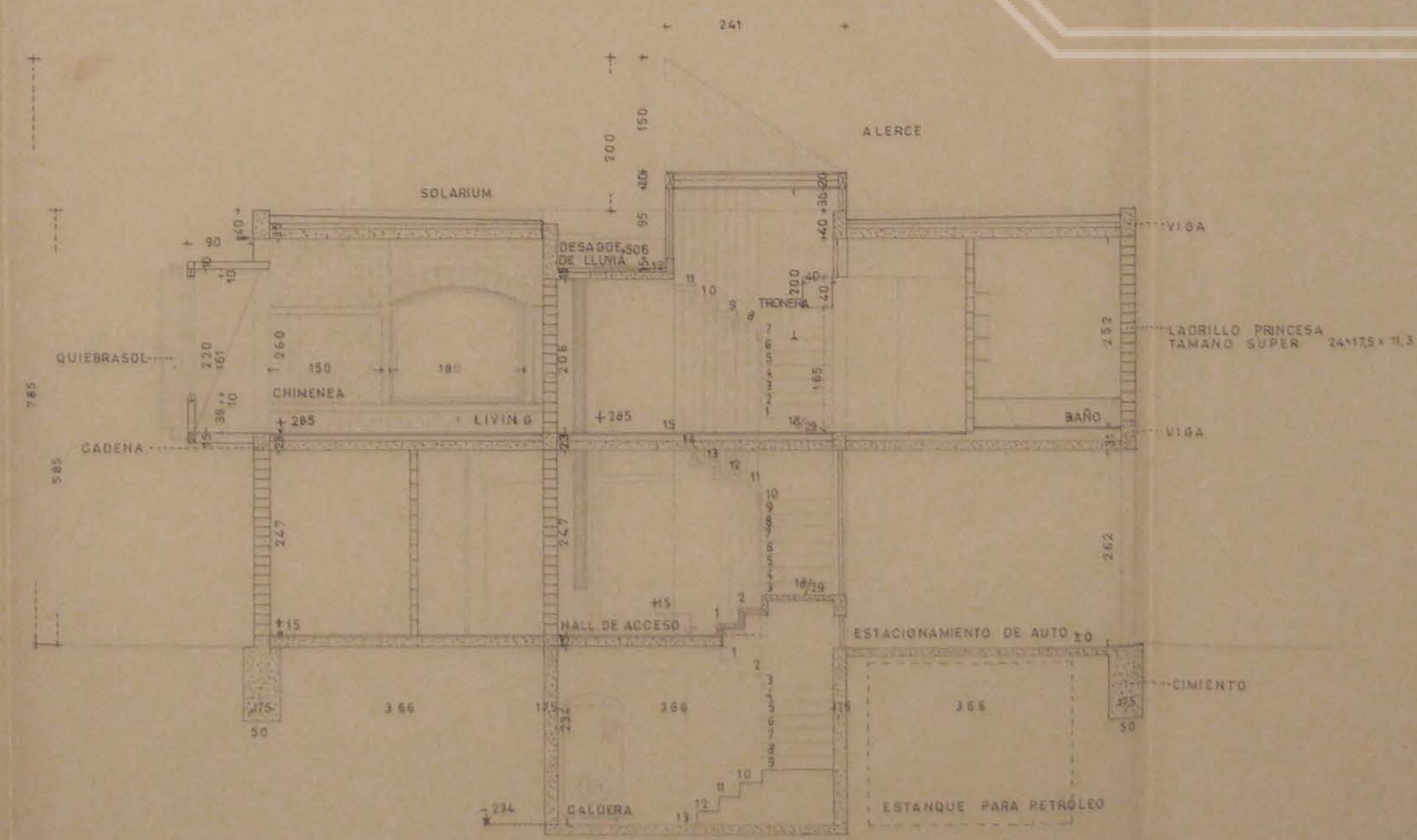
CORTE A-A
