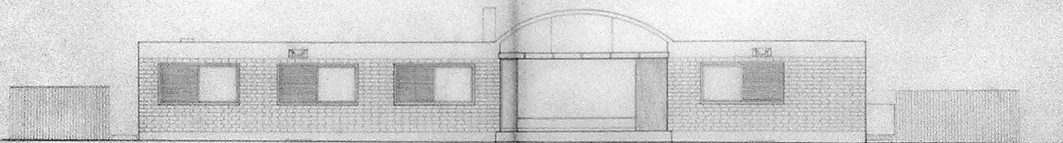
FACHADA NORTE
