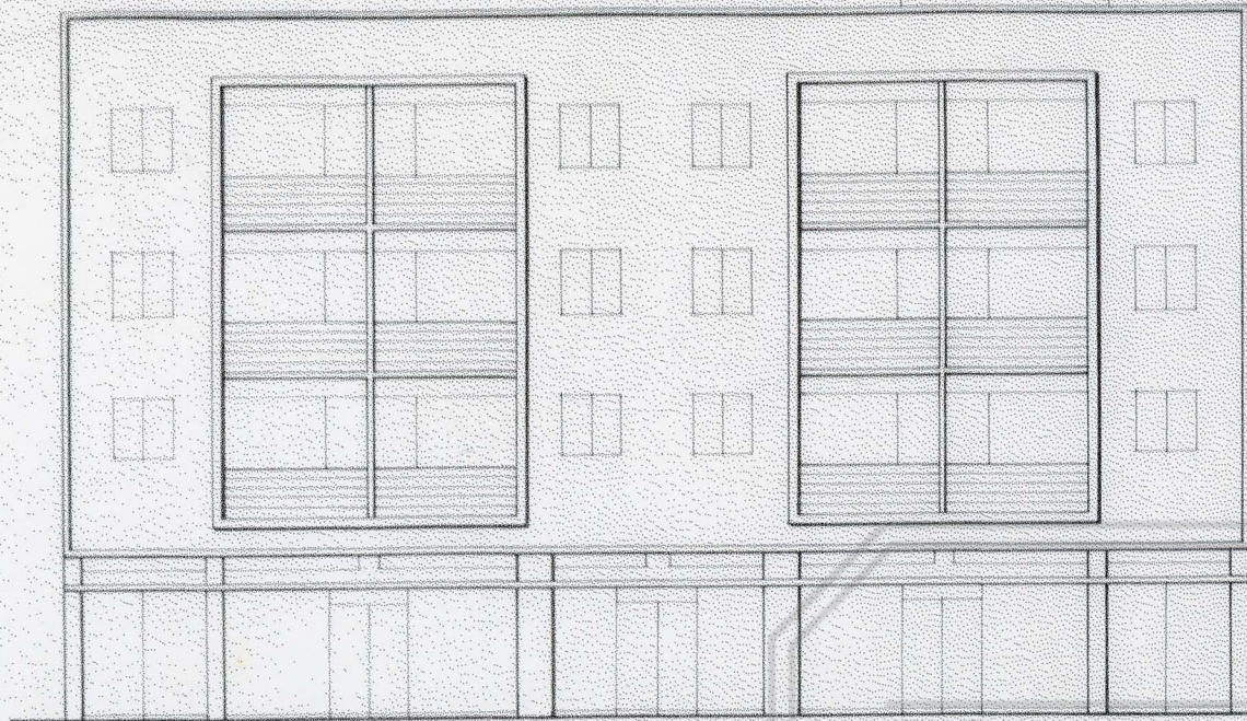
ELEVACION NORTE EDIFICIO DE DEPARTAMENTOS
