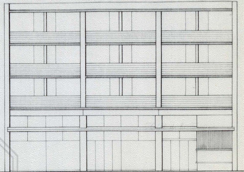
ELEVACION PONIENTE HOTEL
