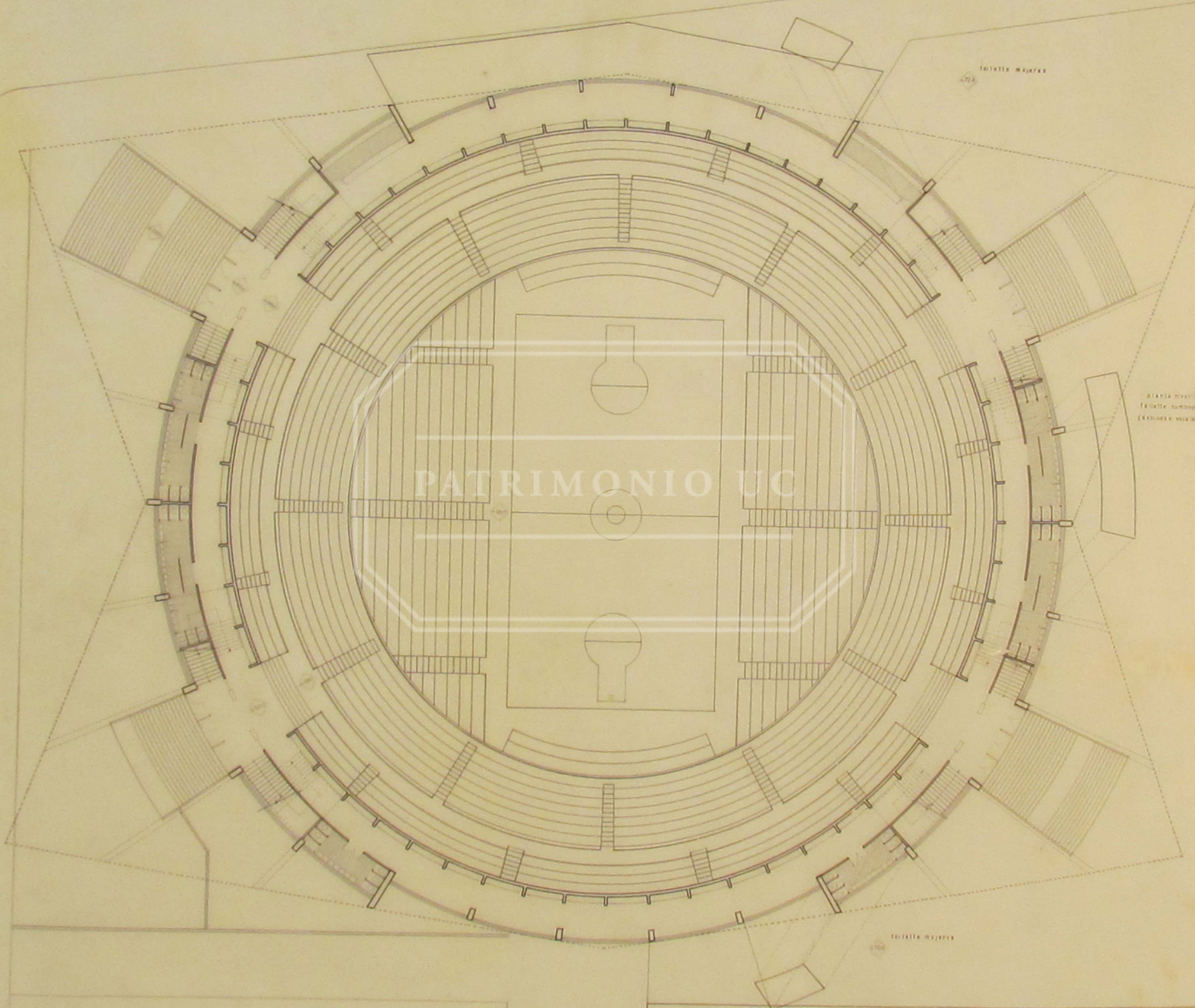
PLANTA A NIVEL DEL BALCON 3 GIMNASIO CUBIERTO MUNICIPAL DE TALCAHUANO ANTEPROYECTO 'MANUTARA'
