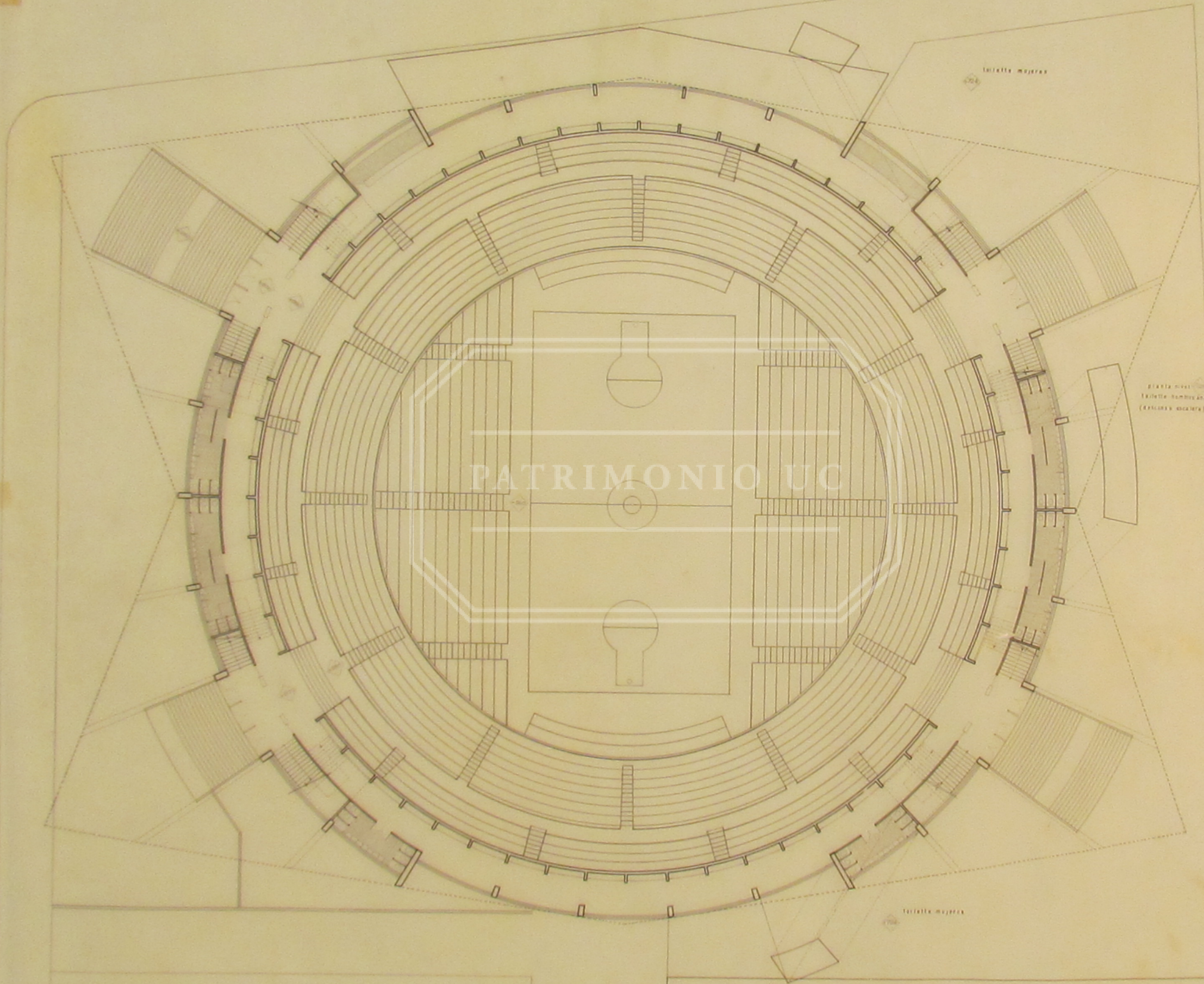
PLANTA A NIVEL DEL BALCON GIMNASIO CUBIERTO MUNICIPAL DE TALCAHUANO ANTEPROYECTO "MANUTARA"
