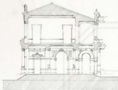
Corte en la entrada
