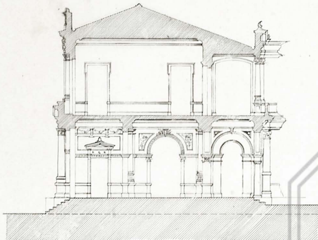
Corte en la entrada
