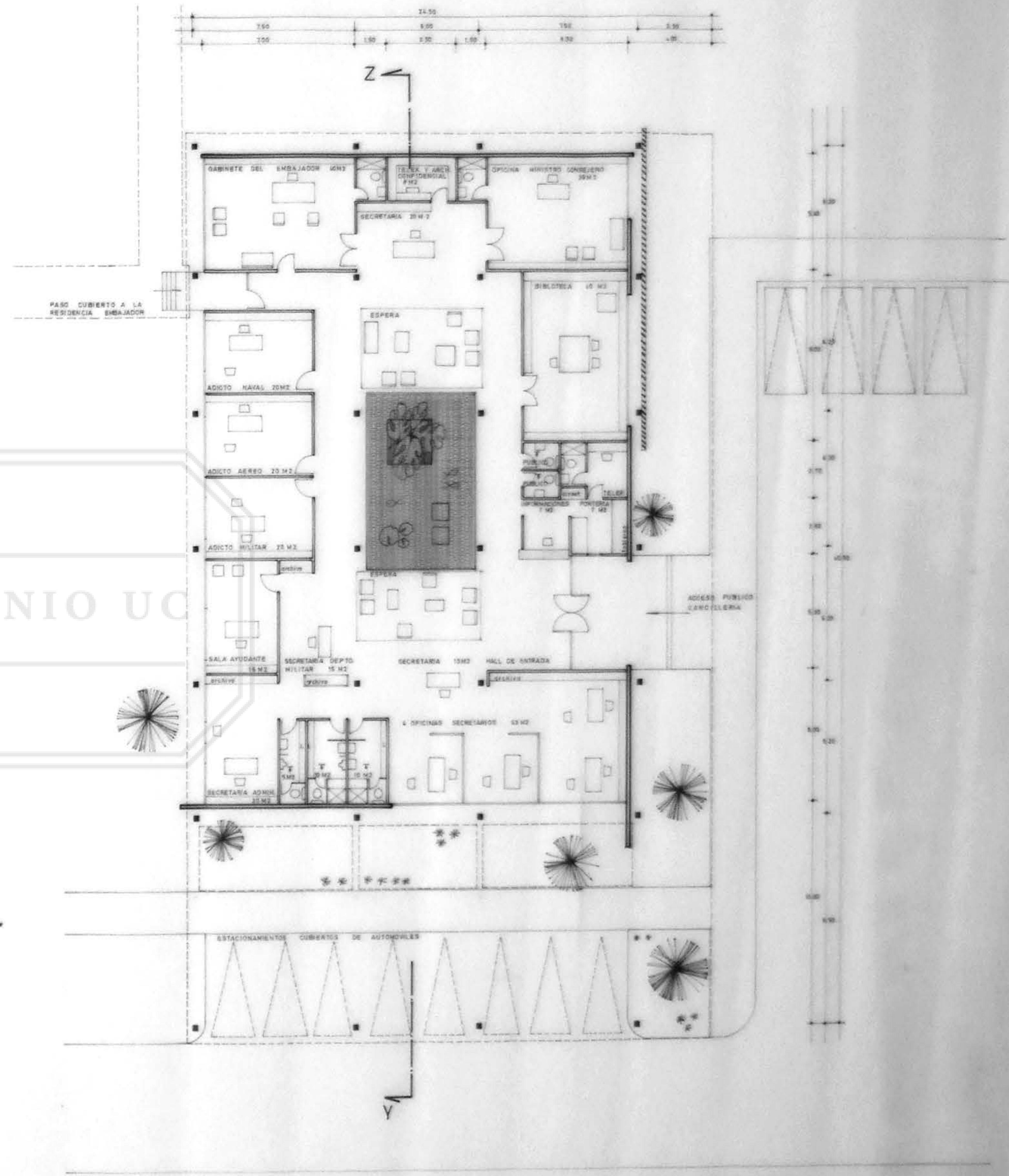
PLANTA CANCELLERIA
