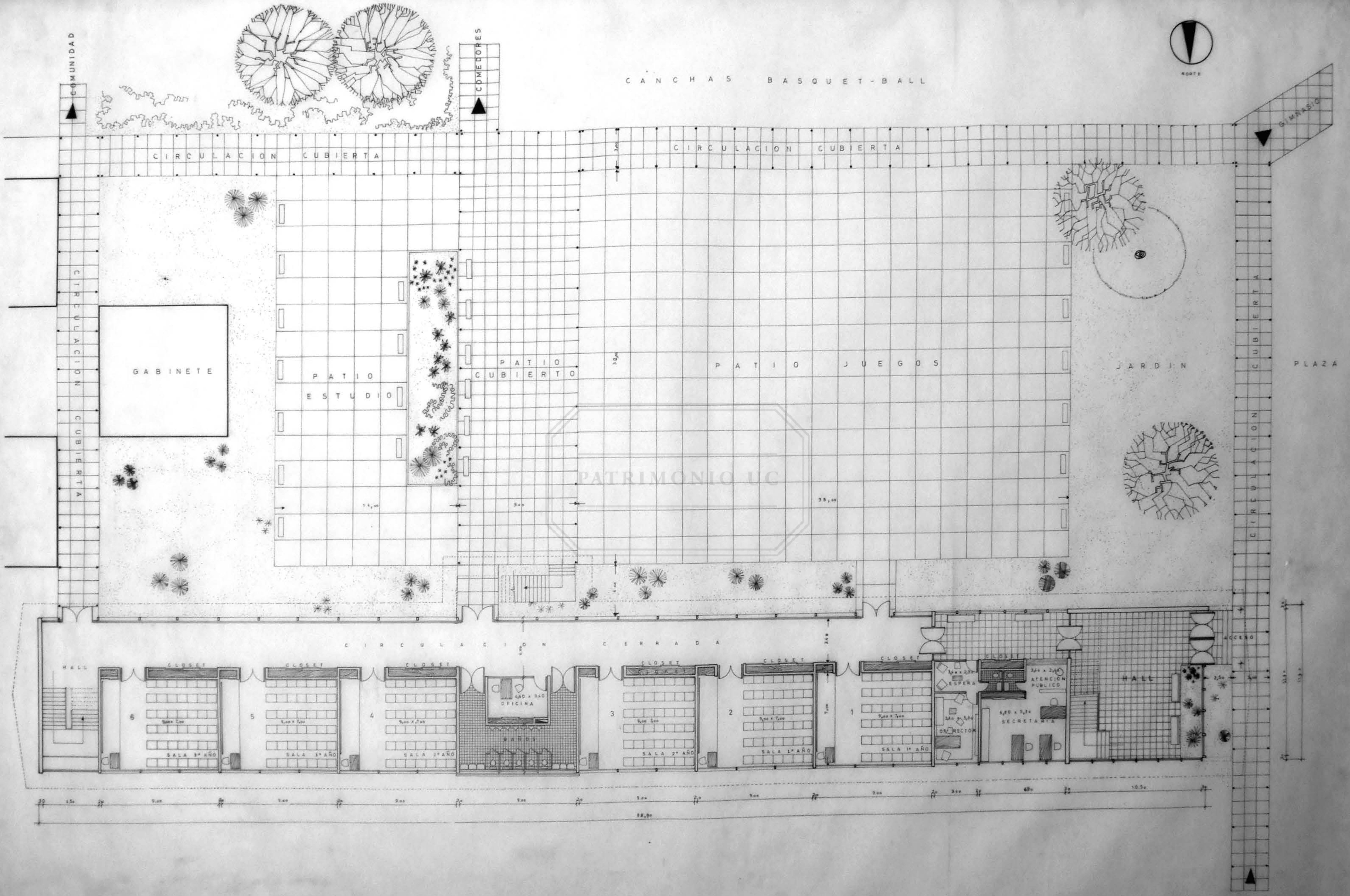
ANTEPROYECTO COLEGIO SAN MATEO — OSORNO | ESCALA 1:100 | SUP. 1º PISO 1057.91 M 2 PLANO PABELLON HUMANIDADES — ADMINISTRACION Y SALAS DE CLASES | ARQUITECTOS ALBERTO RIVERO O. — CARLOS AGUIRRE M.
