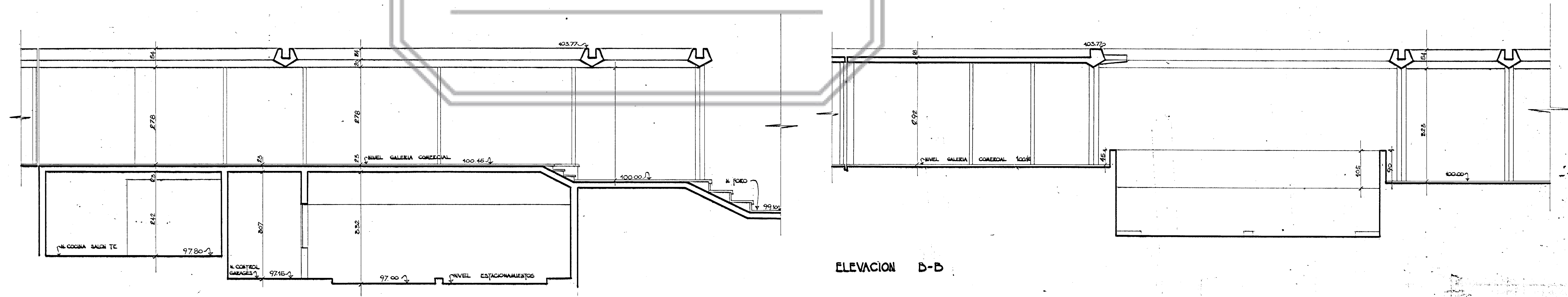
ELEVACION-CORTE D-D
