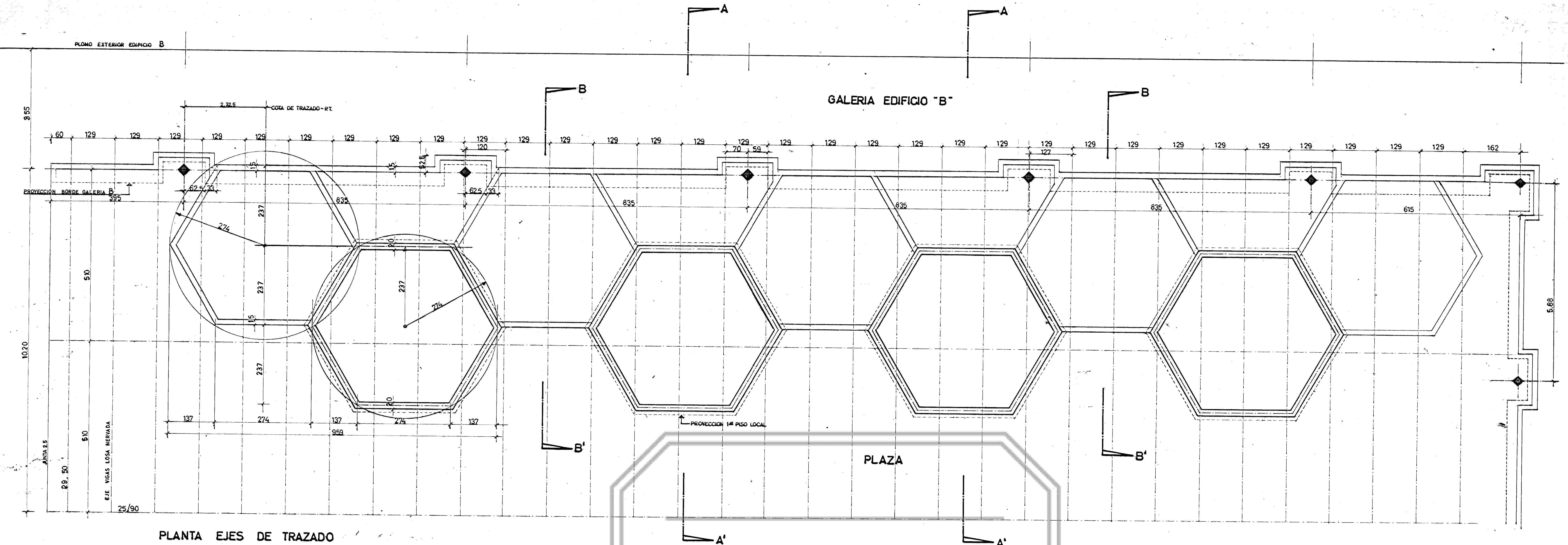
PLANTA EJES DE TRAZADO
