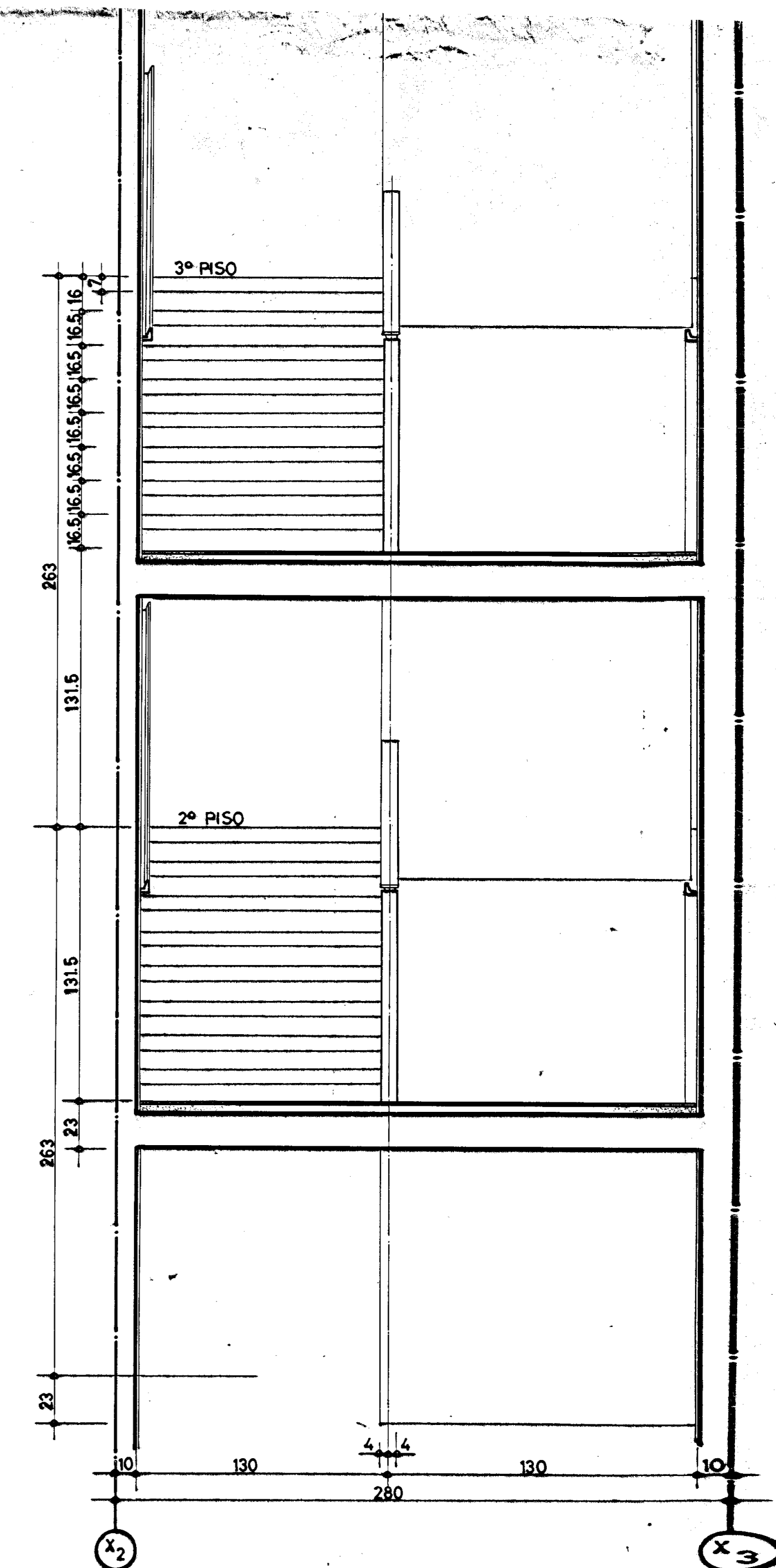
CORTE 4-4
