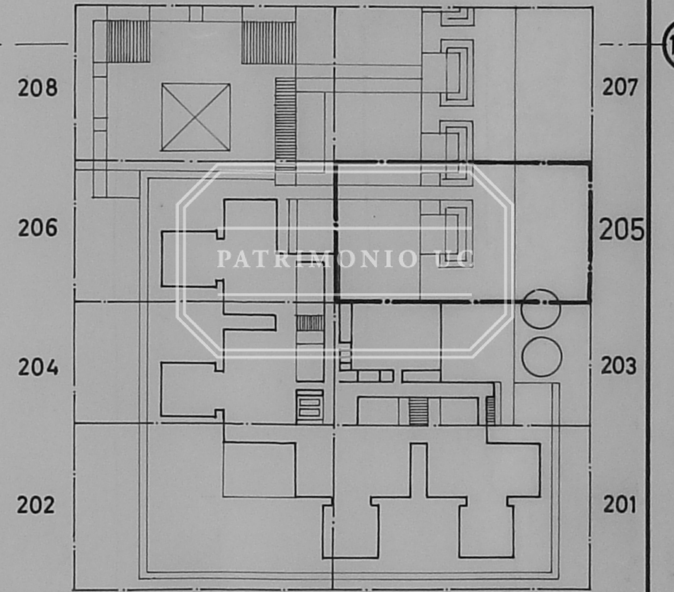
PLANTA SEGUNDO PISO ESC. 1: 1000
