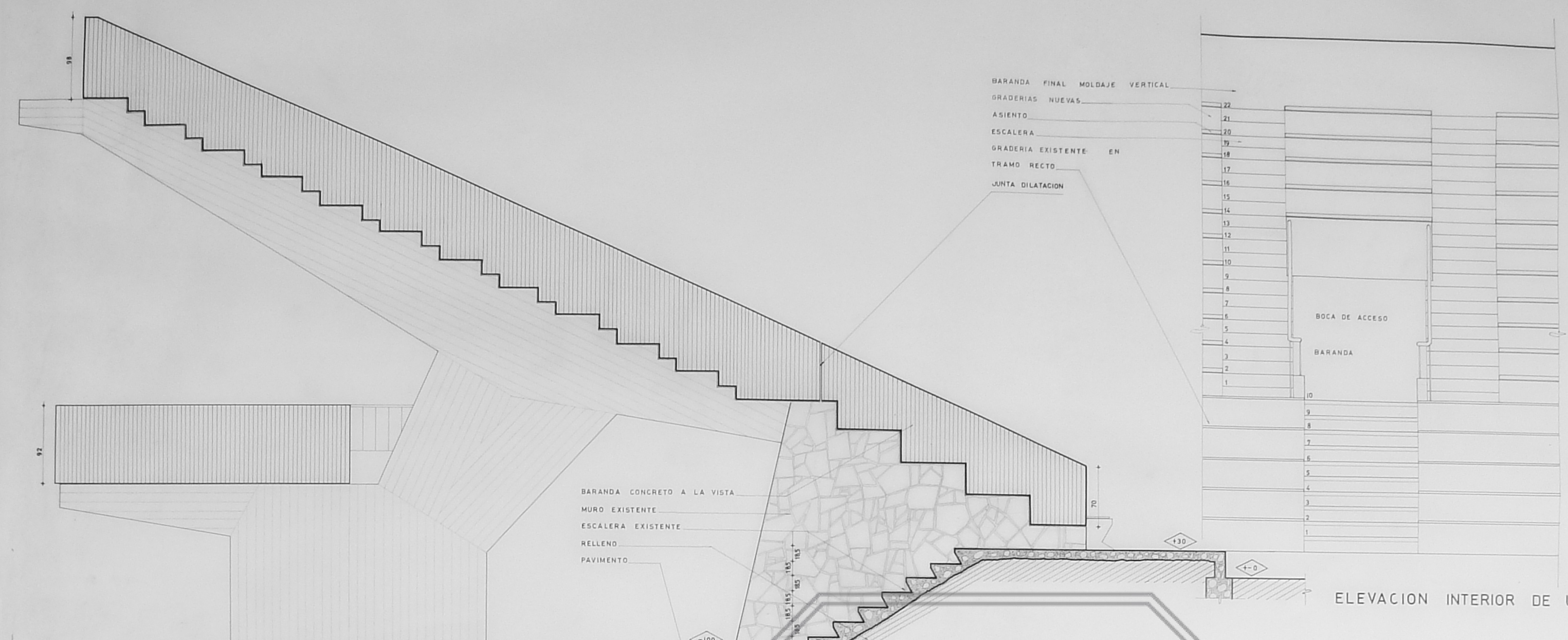
CORTE FF'
