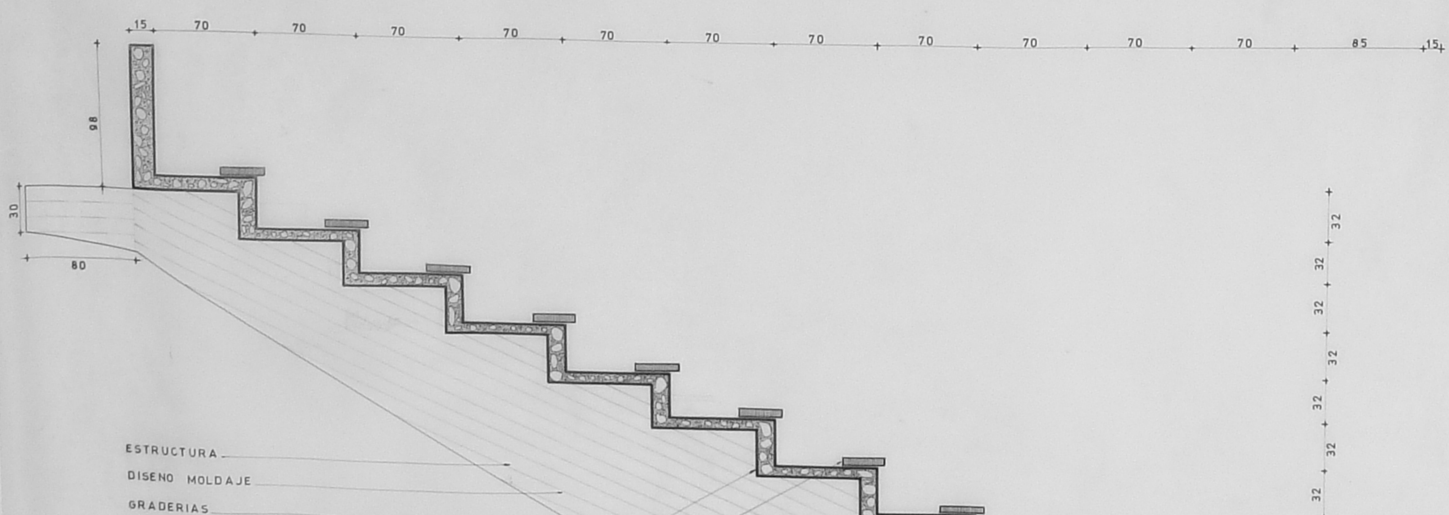
CORTE FF'
