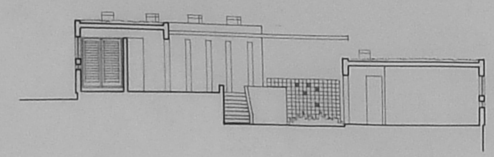
CORTE 2-2
