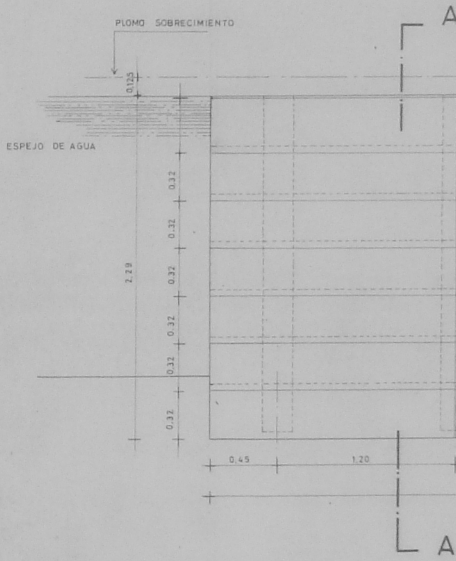
PLANTA esc. 1:20
