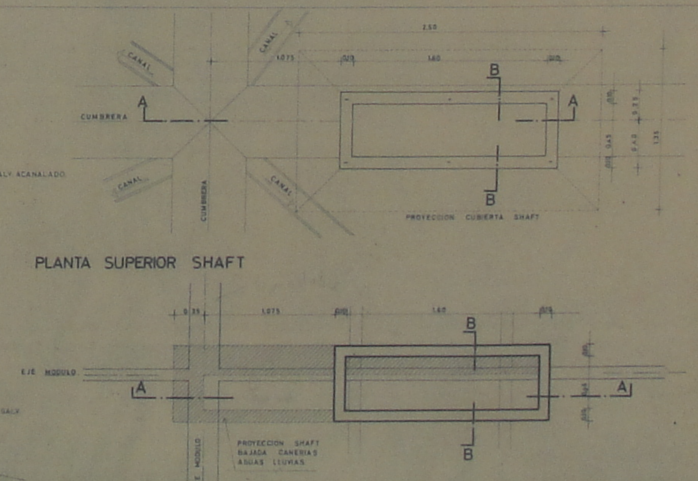
PLANTA EN ENTRETECHO
