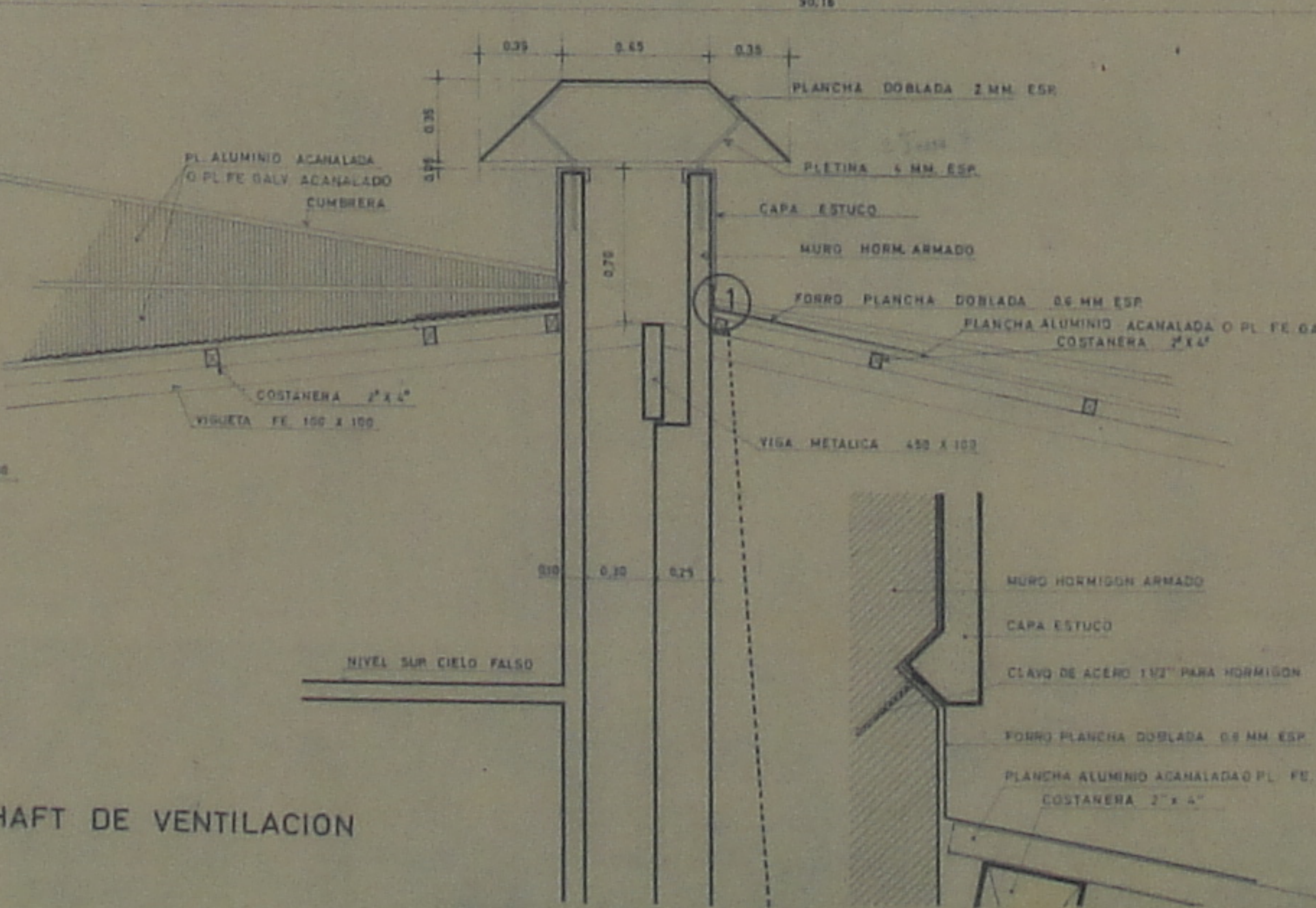
CORTE B-B
