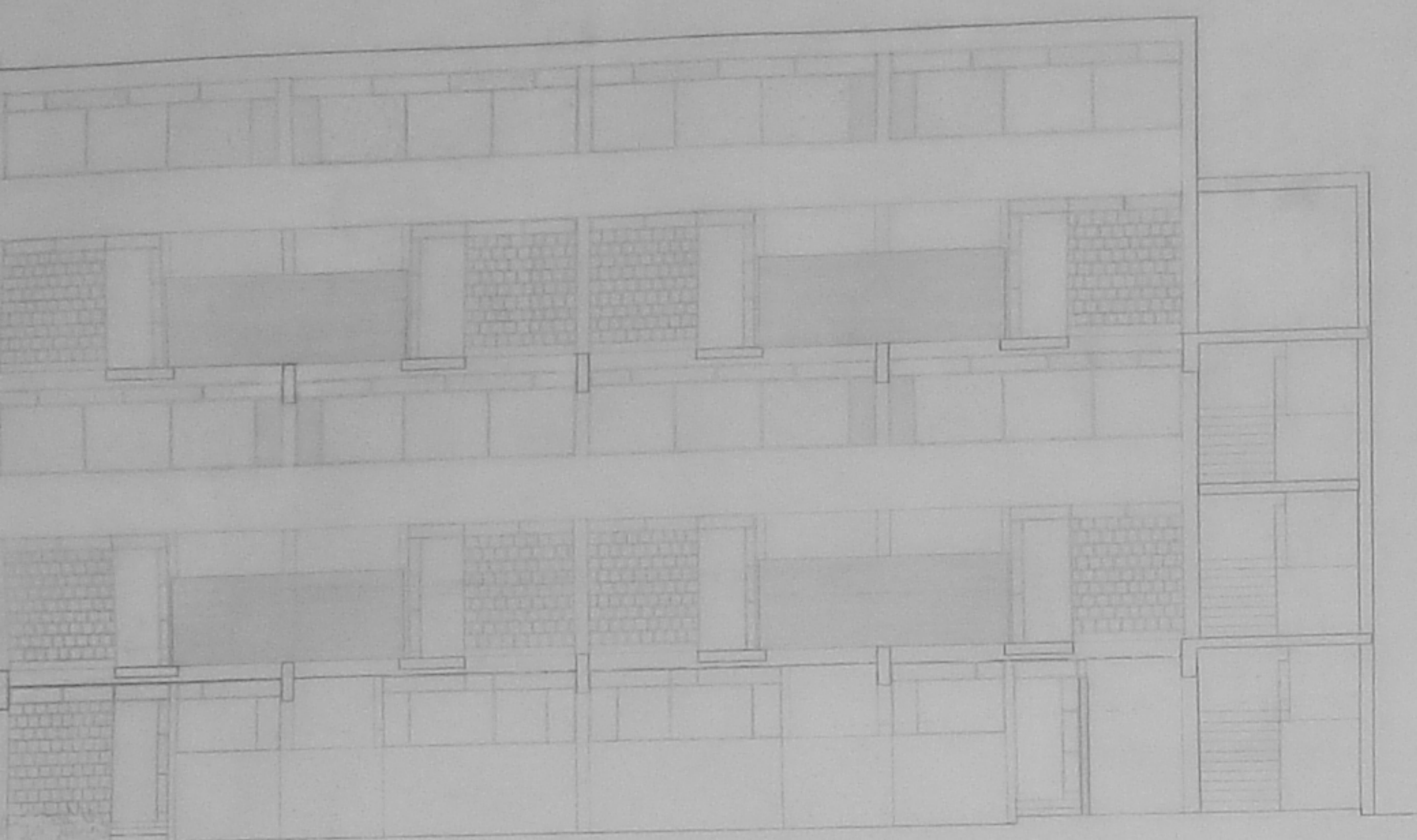
FACHADA SUR SIN BALCON BLOQUES C Y D
