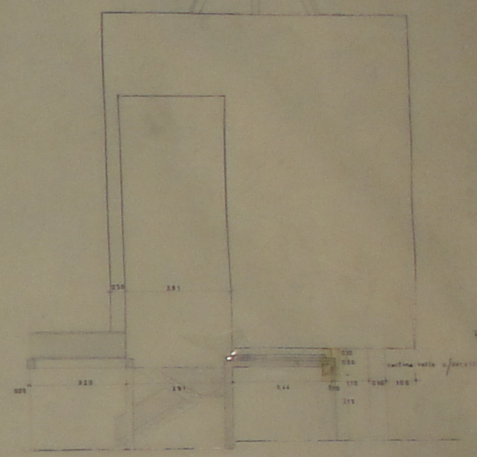
FACHADA ORIENTE BLOQUE B Y CORTE LOCALES
