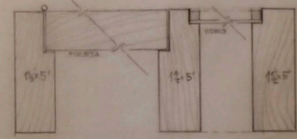
DETALLE TÍPICO DE PUERTAS VENTANAS ESC. 1:15 EXCEPTO LAS 9 - 6 - 2 - 7 CON MARCO 1/2
