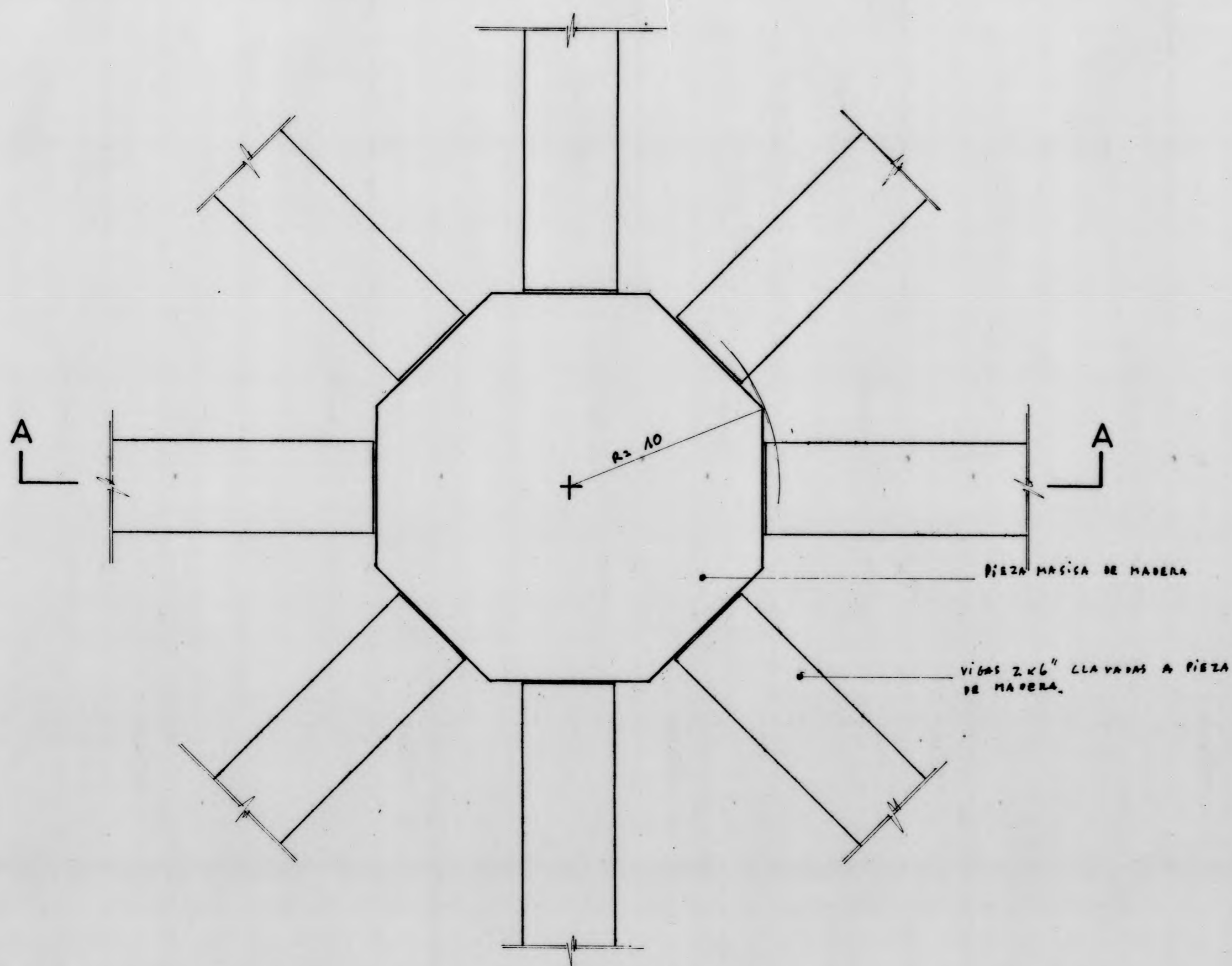
PLANTA ANILLO CENTRAL SUPERIOR ESC. 1:2
