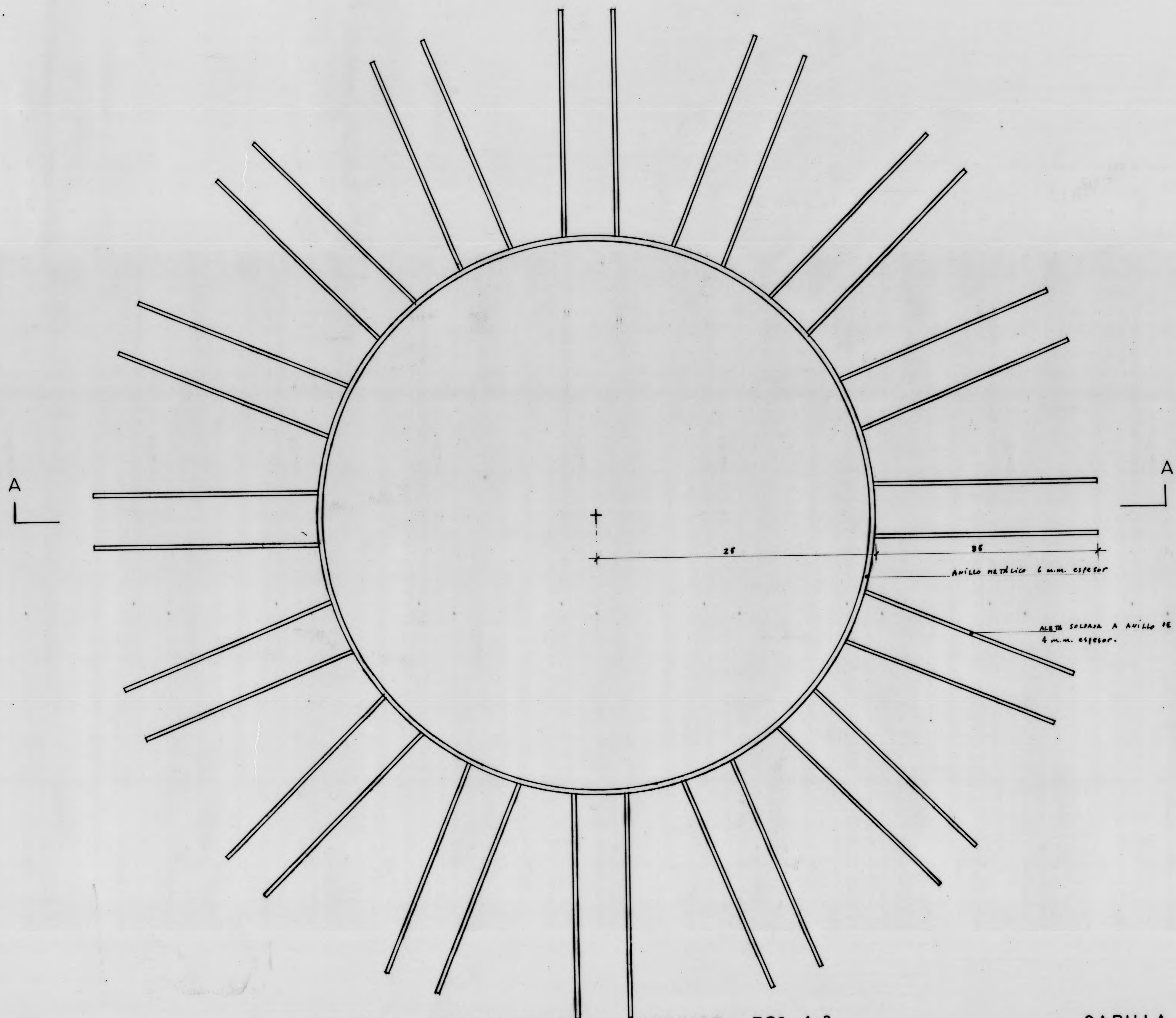
PLANTA ANILLO CENTRAL INFERIOR ESC. 1:2
