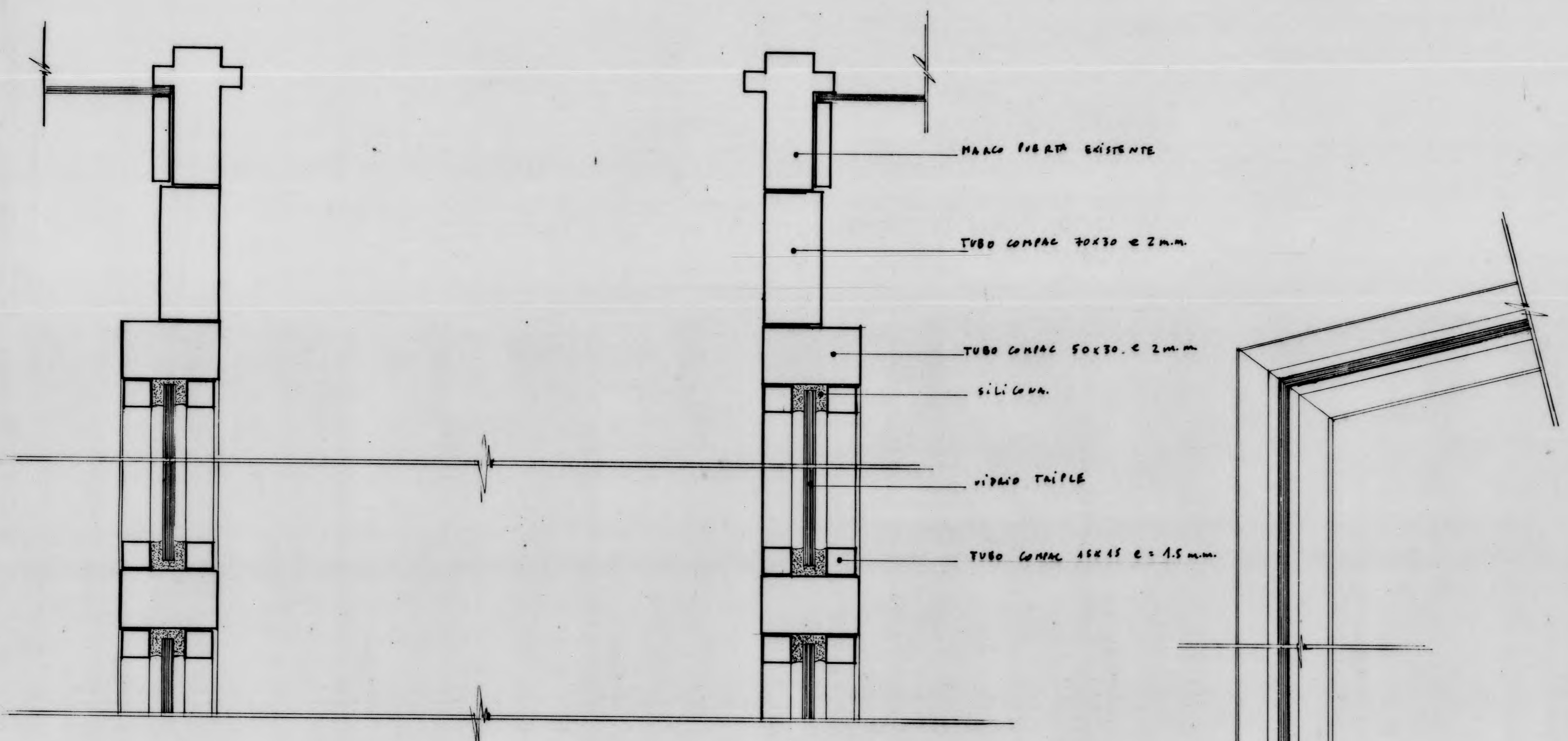
PLANTA DETALLE GALERIA CAPILLA CON EDIFICIO EXISTENTE ESC. 1:2
