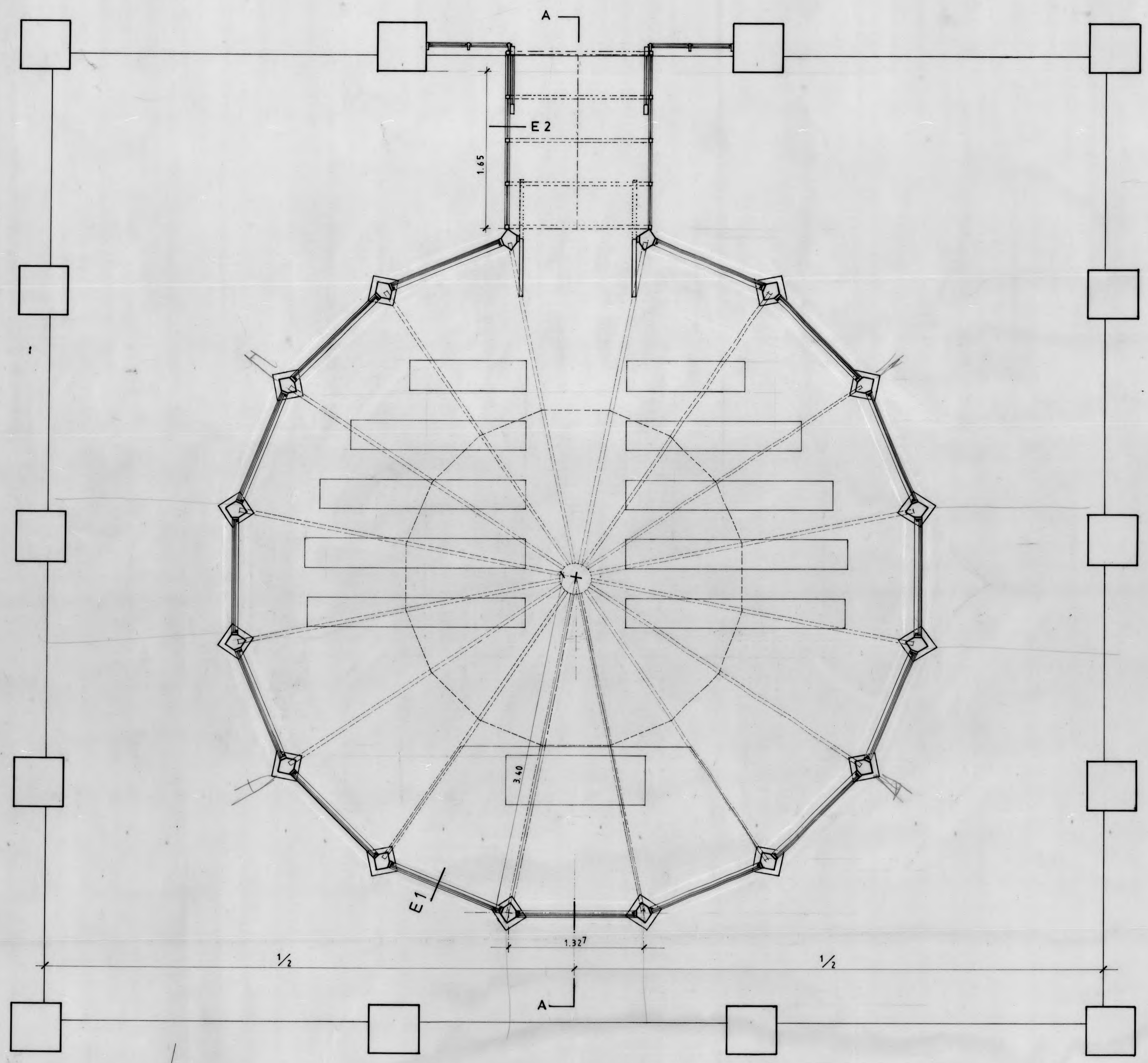
PLANTA ESC. 1:25
