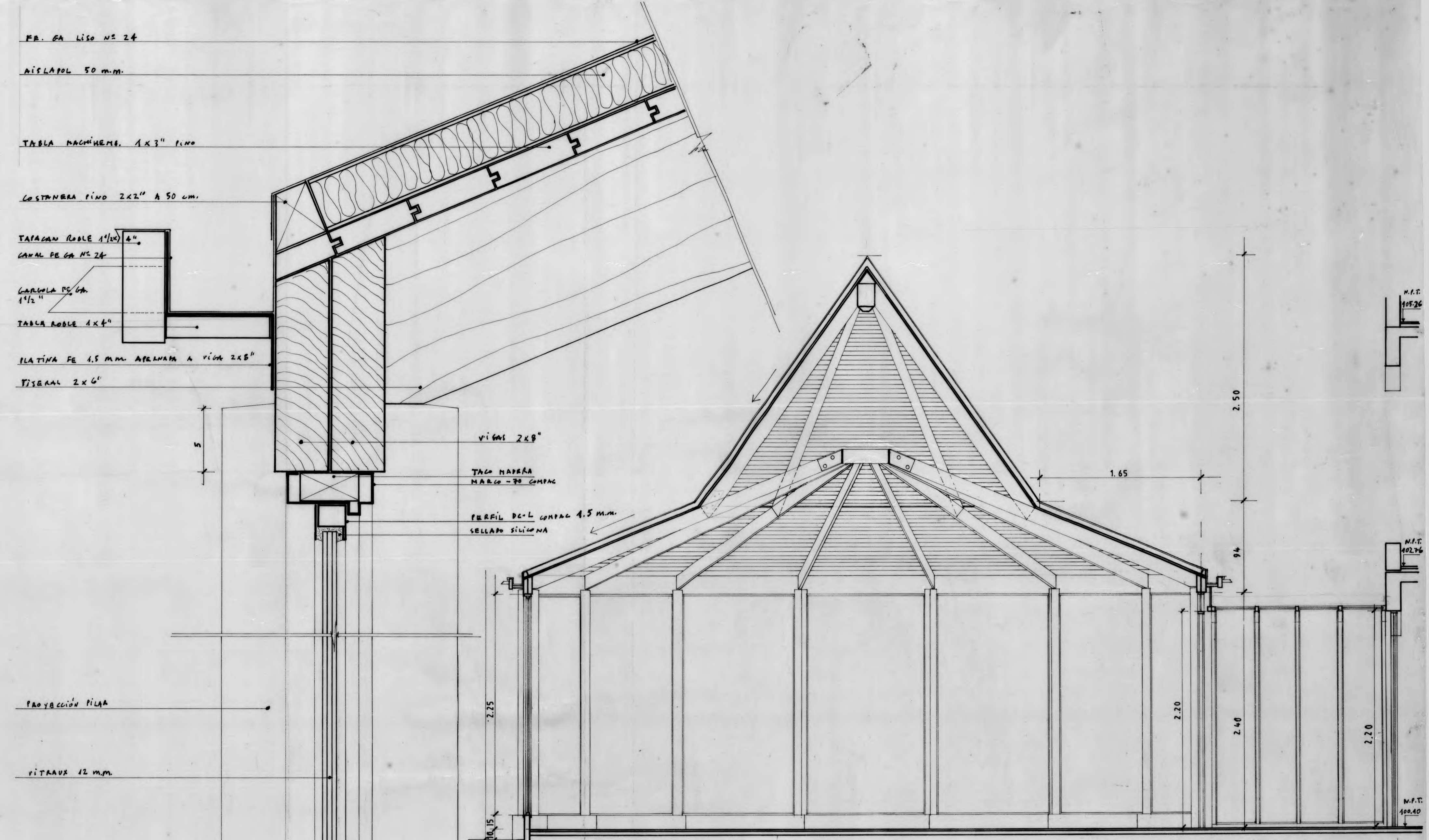
CORTE A-A
