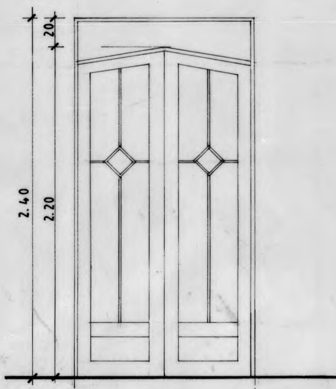
PUERTA DE VAIVEN CAPILLA ESC. 1:25
