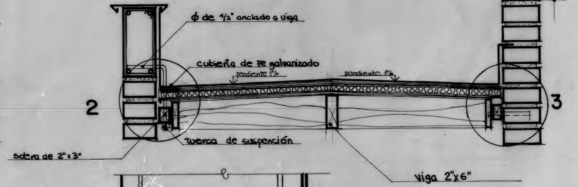
ANCLAJE ENVIGADO TECHUMBRE A MURO (GALERIAS) escala 1:2
